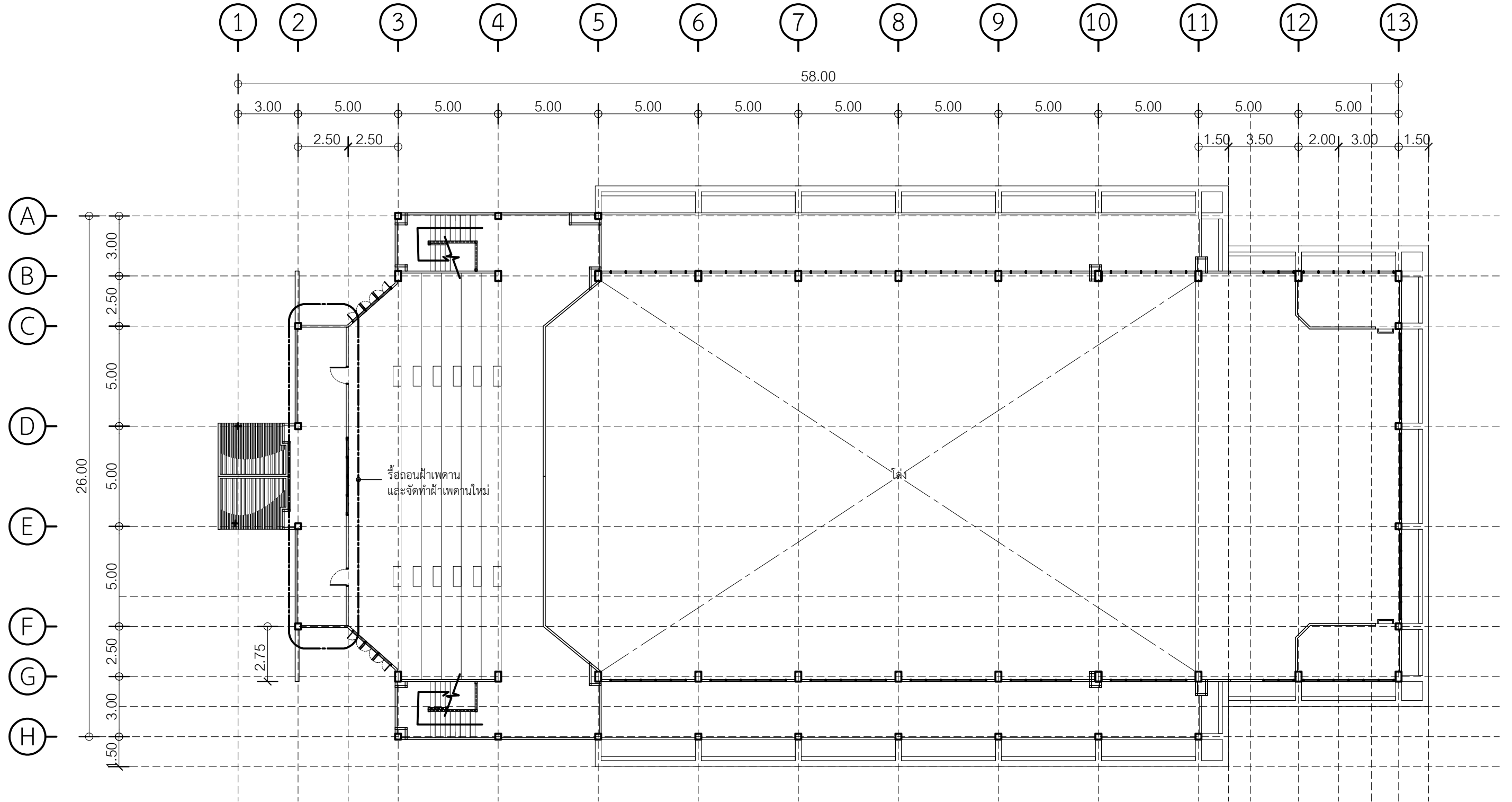
แบบแสดงการรื้อถอนแปลนชั้นลอย มาตราส่วน 1:200
