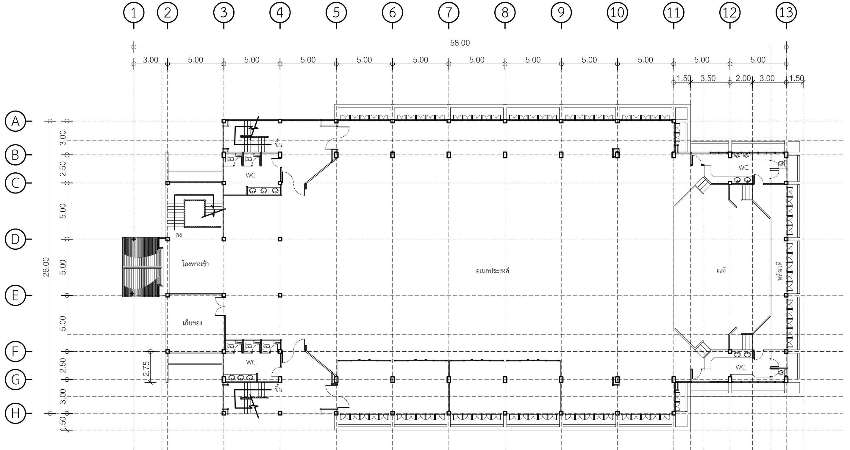
แบบแสดงแปลนชั้นที่ 2 เดิม มาตราส่วน 1:250
