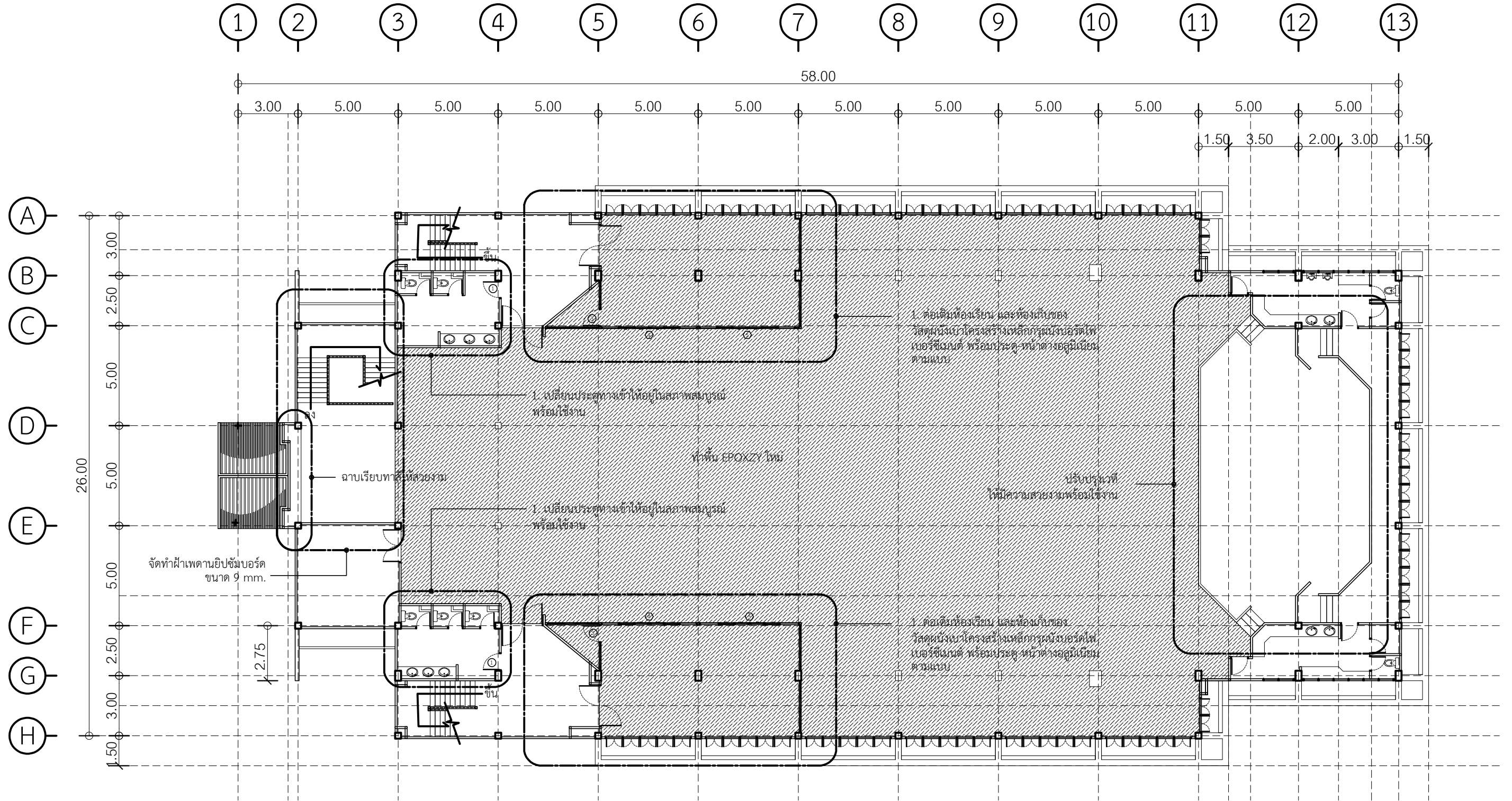
แบบแสดงแปลนชั้นที่ 2 (ปรับปรุง) มาตราส่วน 1:200
