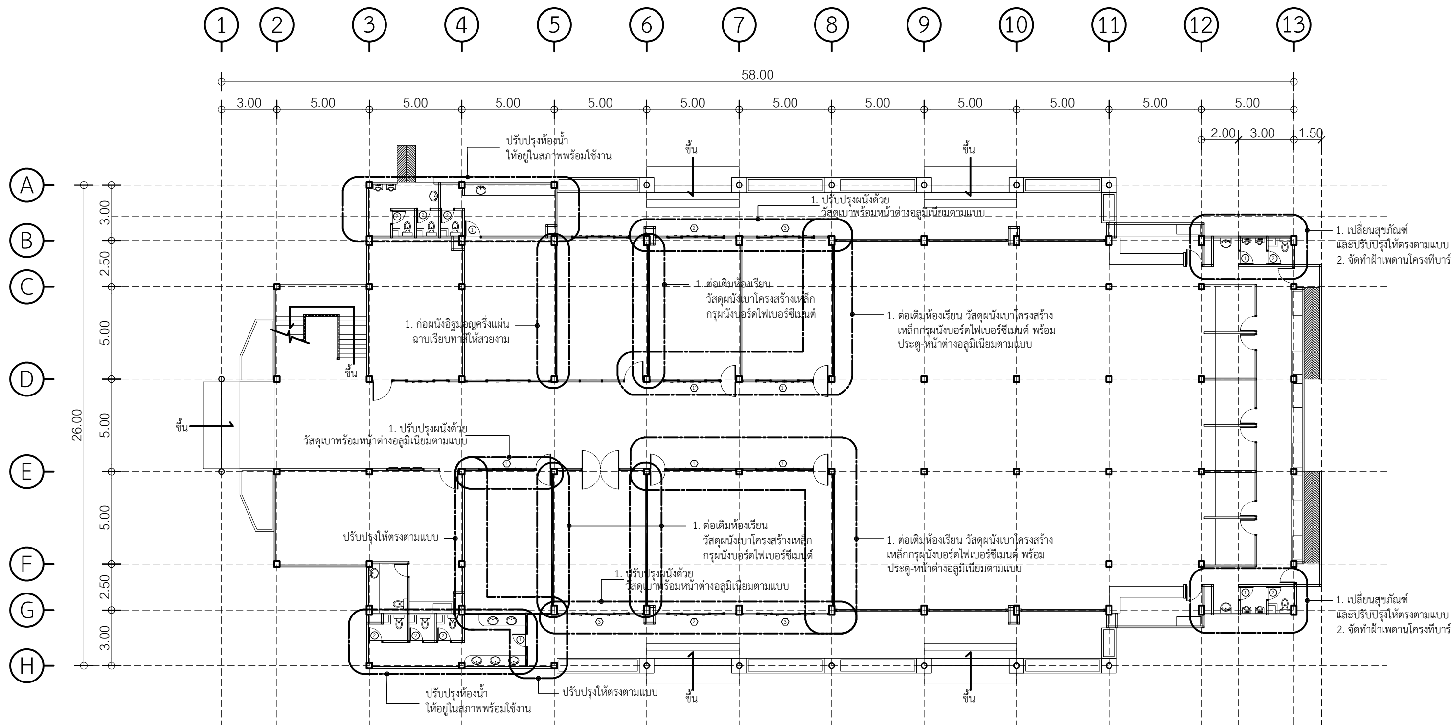
แบบแสดงแปลนชั้นที่ 1 (ปรับปรุง)
