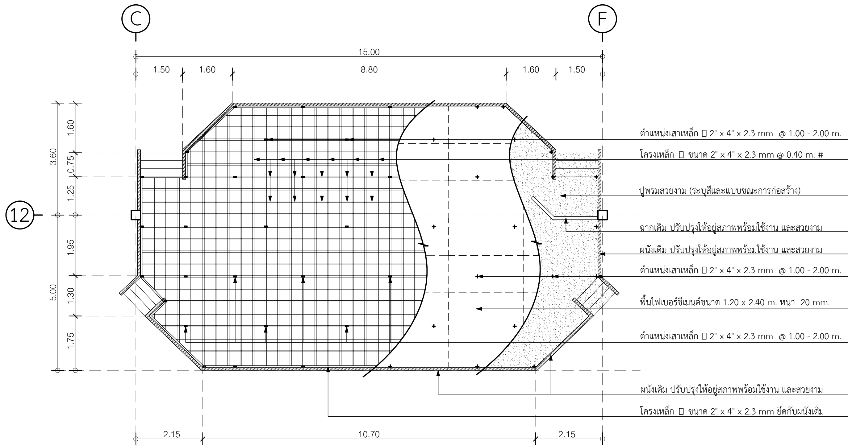
แบบแสดงโครงสร้างพื้นเวที มาตราส่วน 1:75
