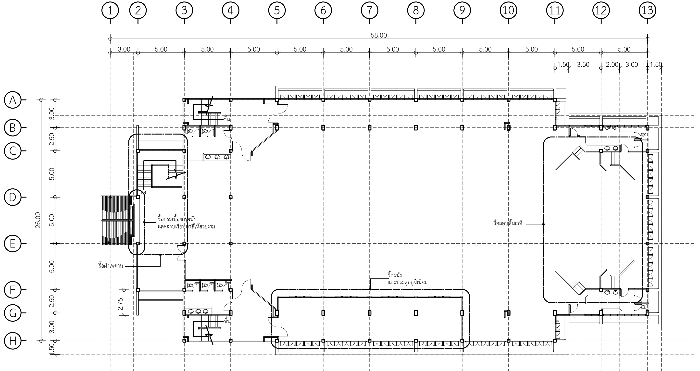
แบบแสดงการรื้อถอนแปลนชั้นที่ 2 มาตราส่วน 1:200
