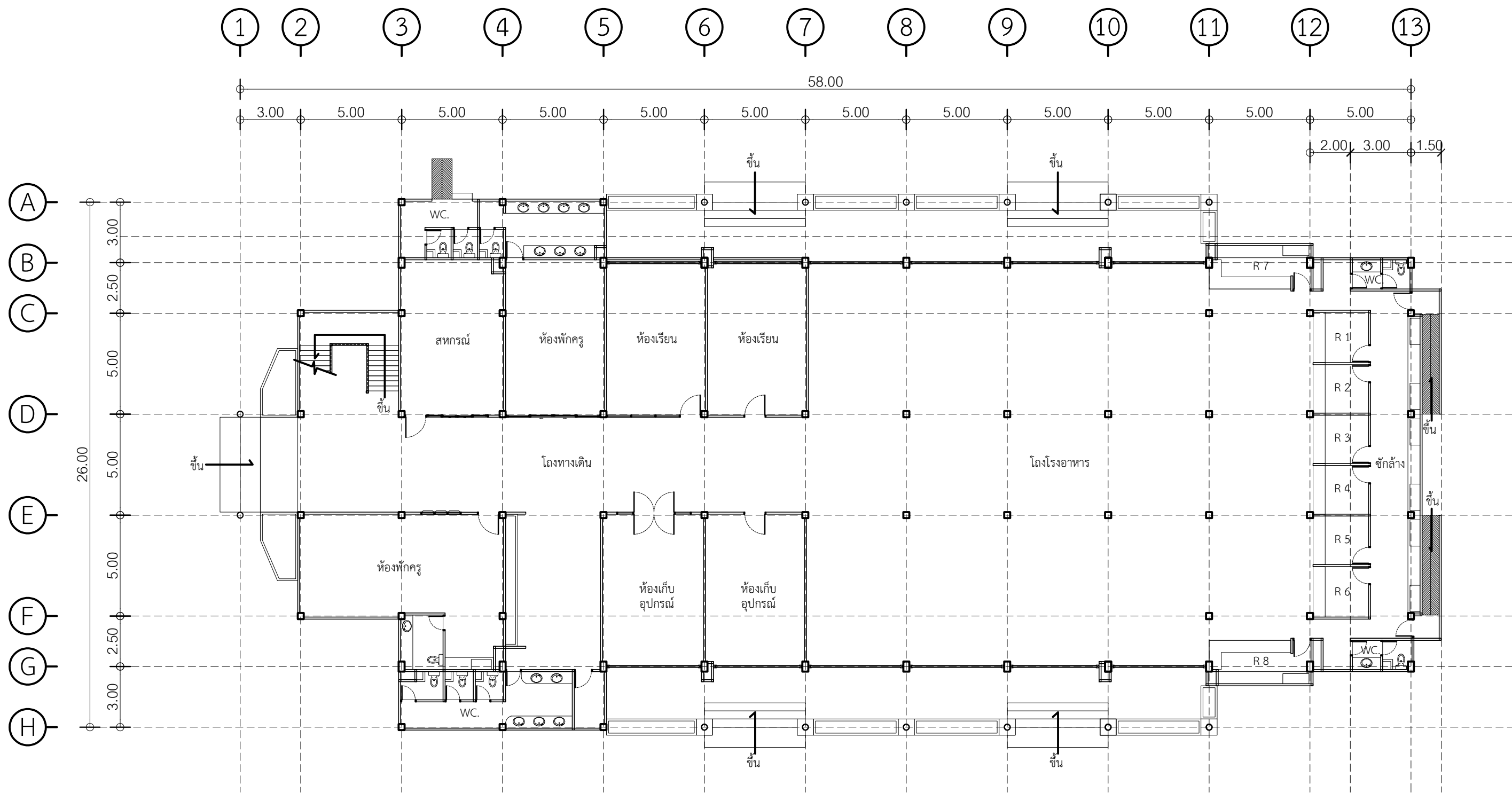
แบบแสดงแปลนชั้นที่ 1 เดิม มาตราส่วน 1:250
