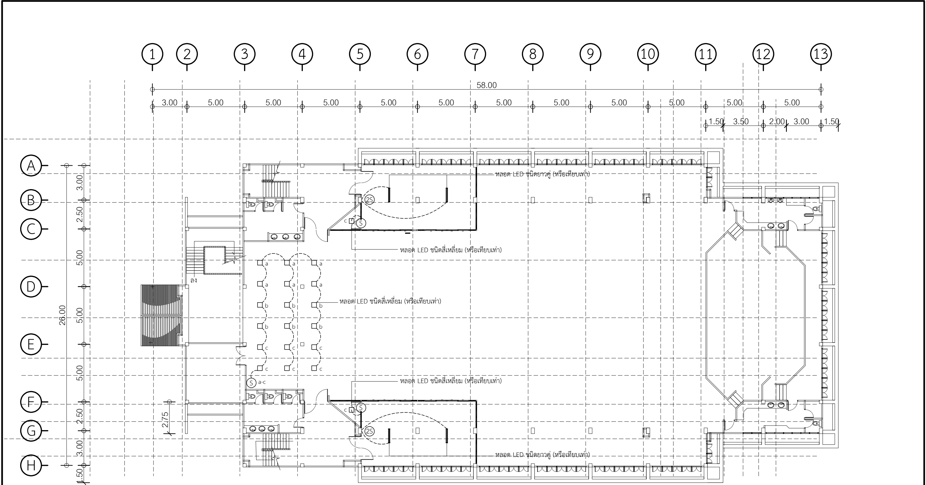
แบบแสดงไฟฟ้าแสงสว่างชั้น 2 ปรับปรุง มาตราส่วน 1:200
