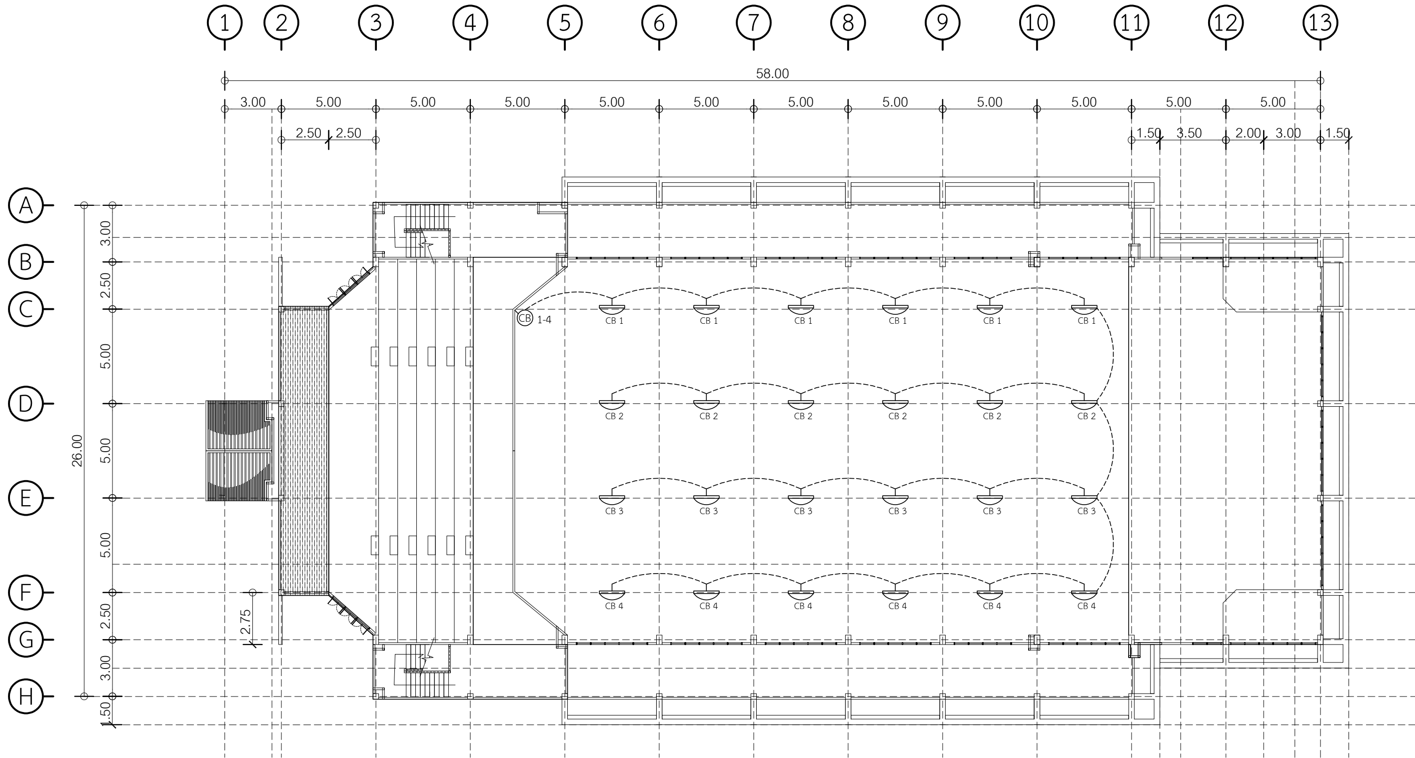
แบบแสดงไฟฟ้าแสงสว่างชั้นลอย ปรับปรุง มาตราส่วน 1:200
